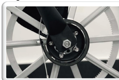
eegoBeltBrake Bandbremse
